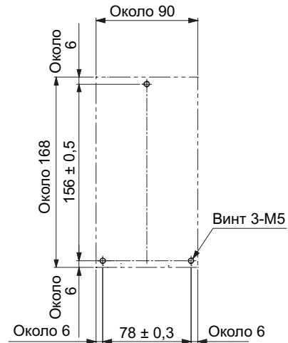
Чертеж для обработки монтажного отверстия
